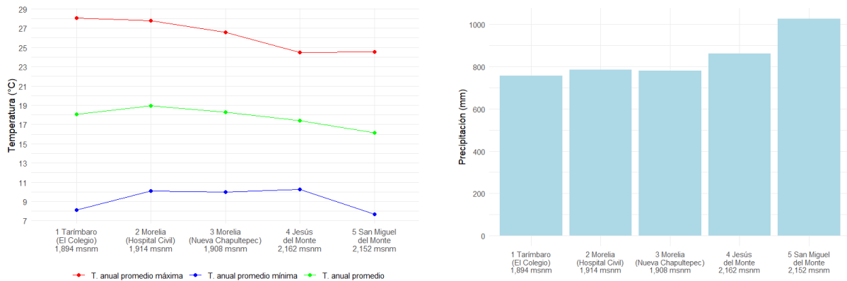
Figura 11. Temperaturas anuales promedio y precipitación acumulada promedio anual por caseta climática
