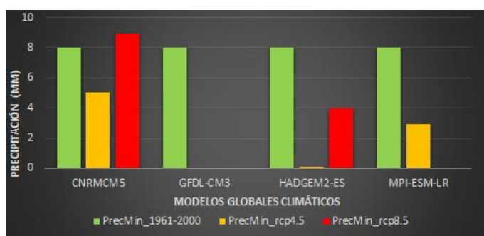
Figura 18. Escenario cercano (2015-2039) para la precipitación mínima con base en el climograma 1981-2010
