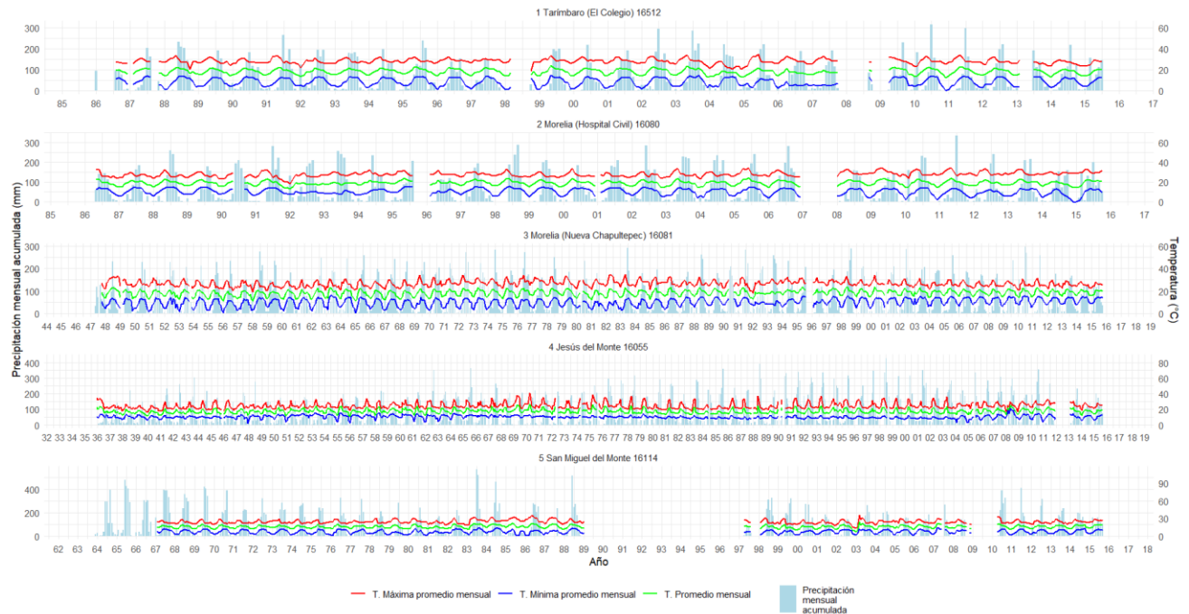
Figura 9. Series de tiempo de precipitación mensual acumulada, temperatura promedio mensual máxima y temperatura promedio mensual mínima
