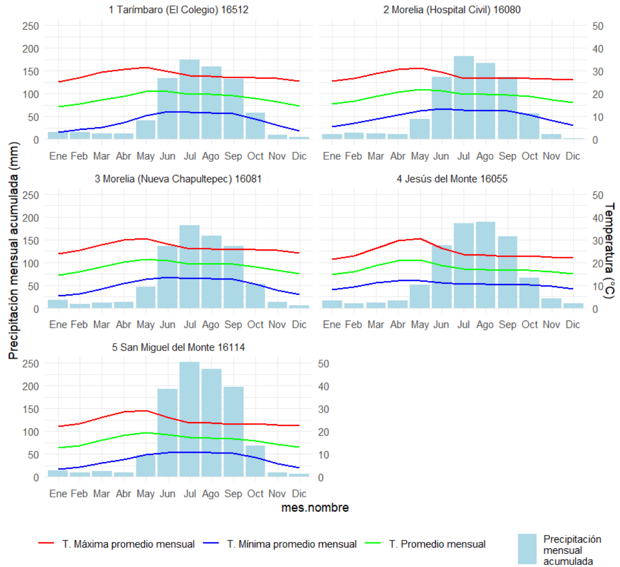
Figura 10. Climogramas de las estaciones climáticas de 1963 a 2015
