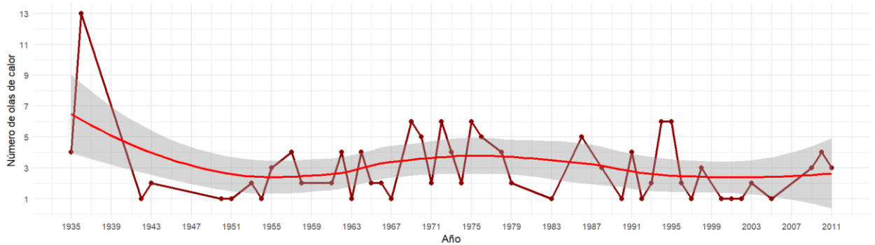
Figura 19. Olas de calor de 1935-2011
