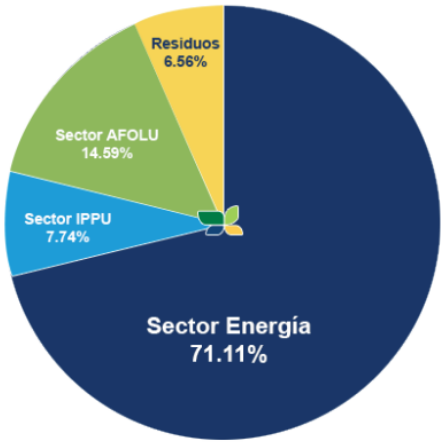
Figura 3. Emisiones GEI en México, 2015
