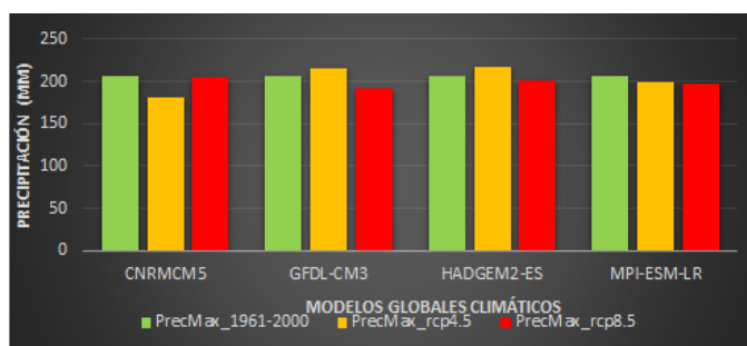
Figura 17. Escenario cercano (2015-2039) para la precipitación máxima con base en el climograma 1981-2010
