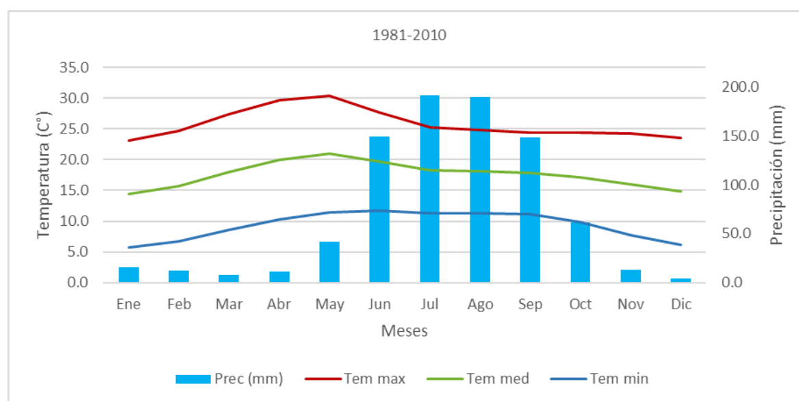
Figura 7. Climograma del municipio de Morelia, (1981-2010).
