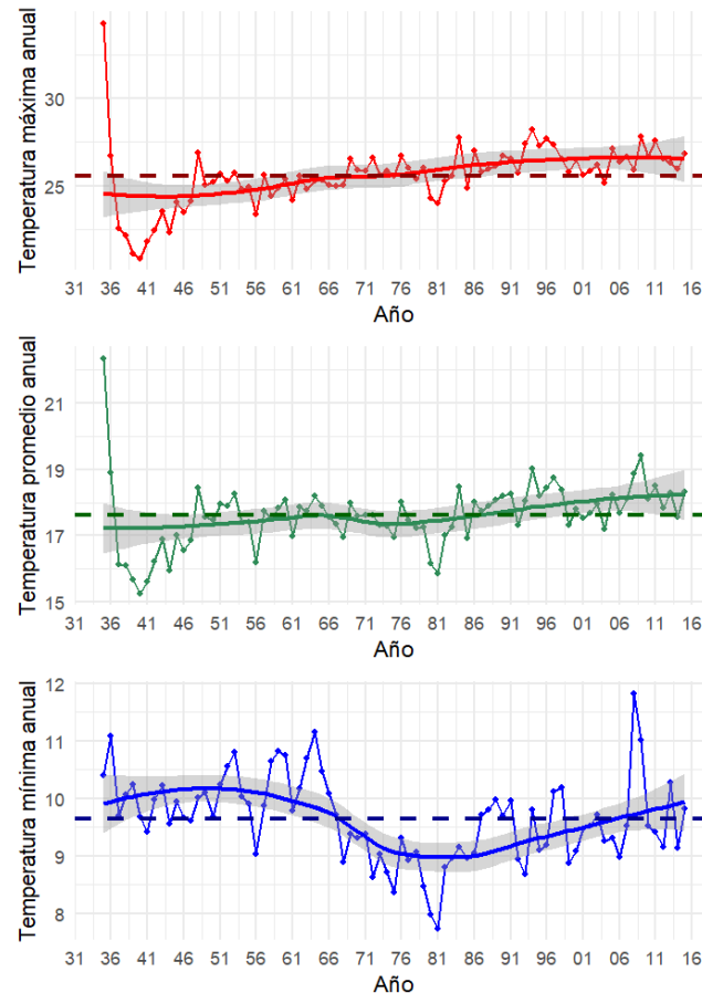
Figura 12. Tendencias de temperaturas promedio anuales de 1935 a 2015
