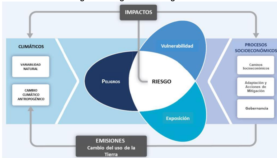
Figura 5. Riesgo climático según el IPCC
