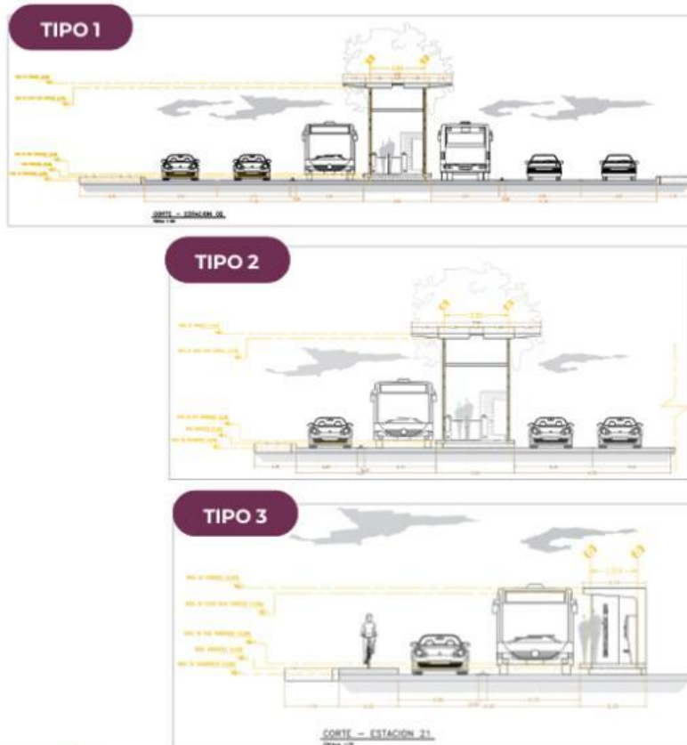
Figura 2-2. Esquema de los tres tipos de estaciones a usar en el proyecto.
