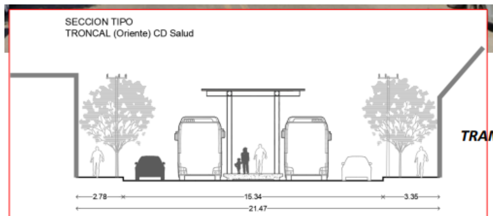
Figura 2-6. Sección del proyecto Troncal B (Oriente). Fuente: Elaboración propia.
